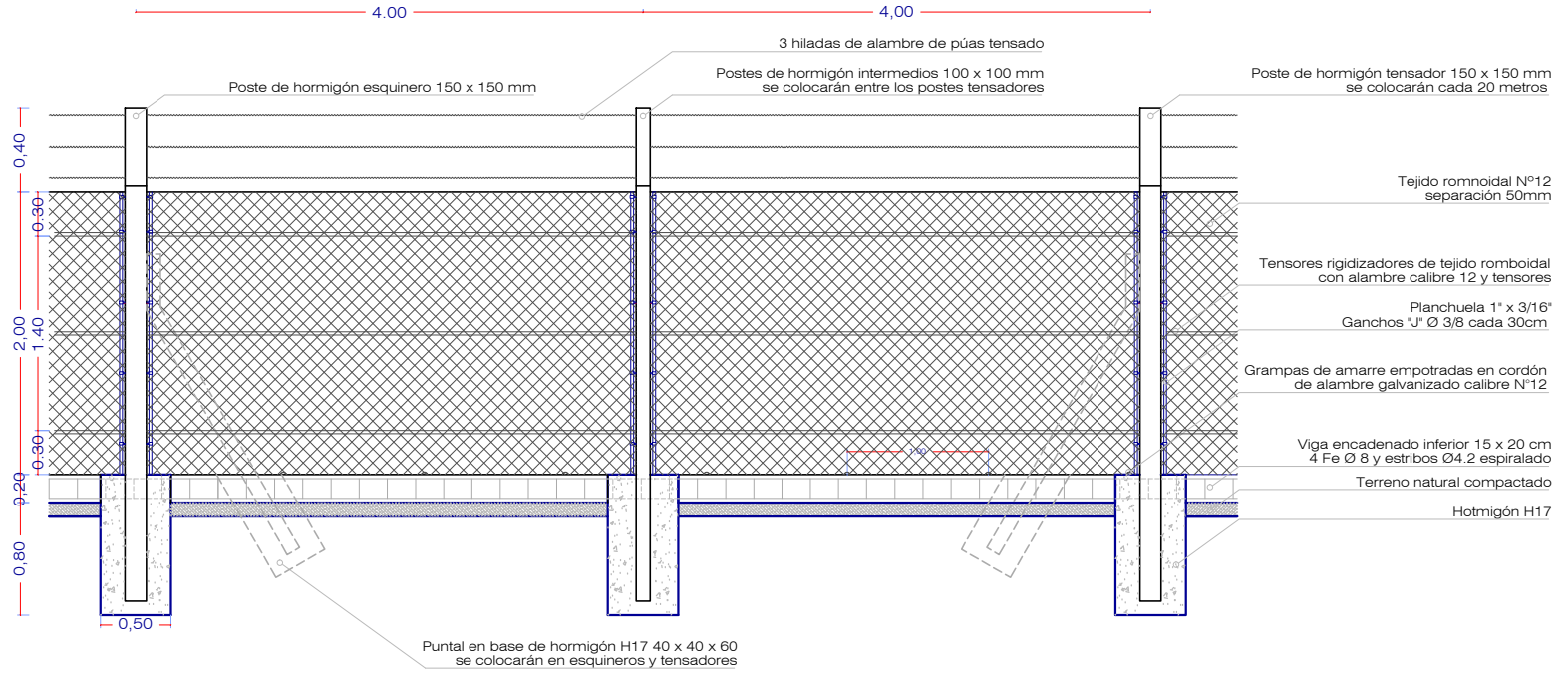
Detalle cerco perimetral olímpico
