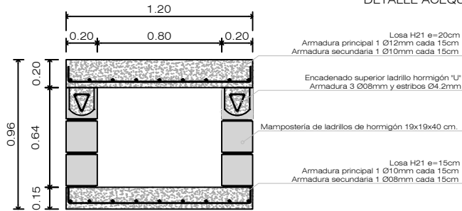
Detalle sección acequia Esc 1:5
