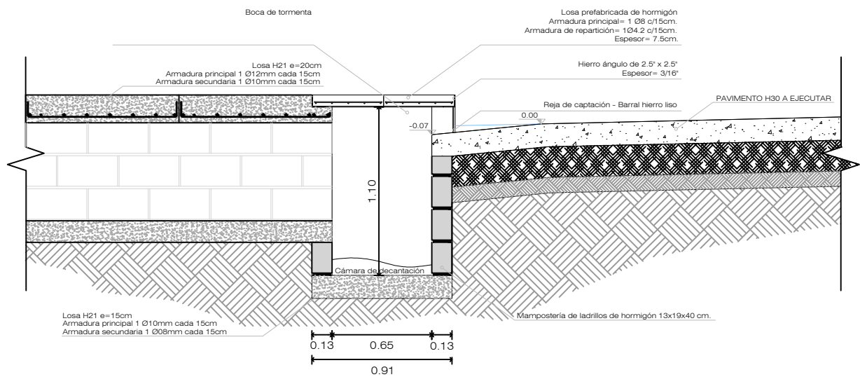
Detalle en perspectiva acequia
