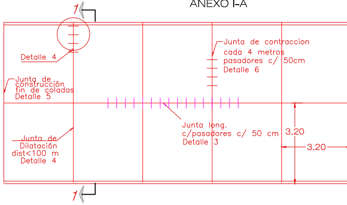
CORTE 1 - 1
