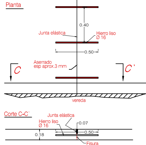
JUNTA DE CONTRACCIÓN CON PASADORES
