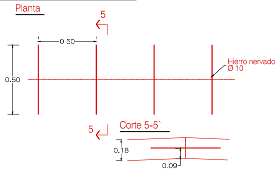
JUNTA LONG. DE CONTRACCIÓN
