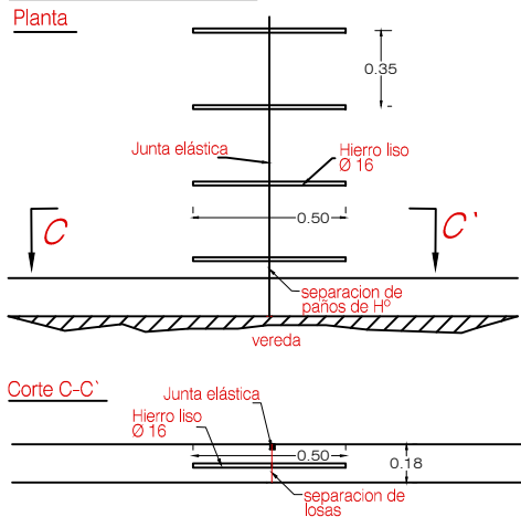
JUNTA DE CONSTRUCCIÓN
