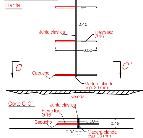
DETALLE 6
